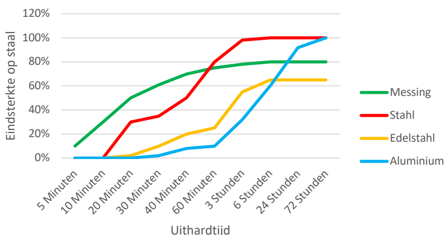
Uithardsnelheden/Schroeven M10
